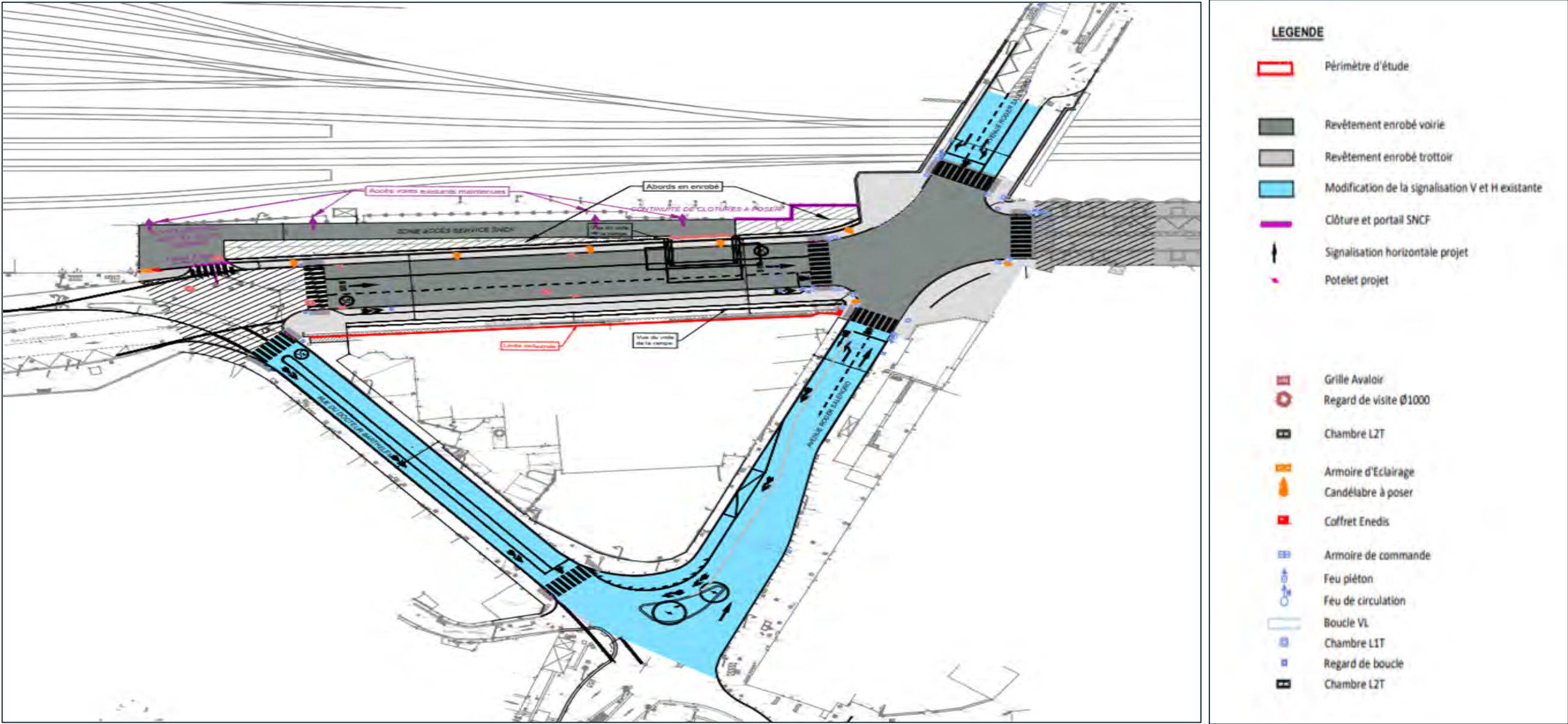
Figure 10 - Plan de masse de la rampe d'accès au PEM d'Aubagne
