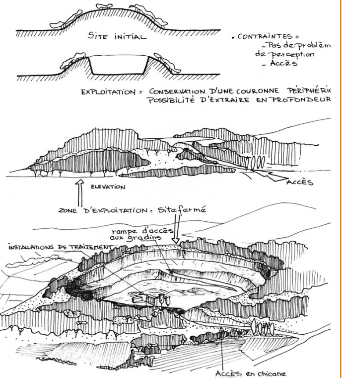
Carrière en puits, schéma de principe
