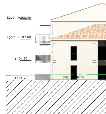
ELEVATION NORD MM -
