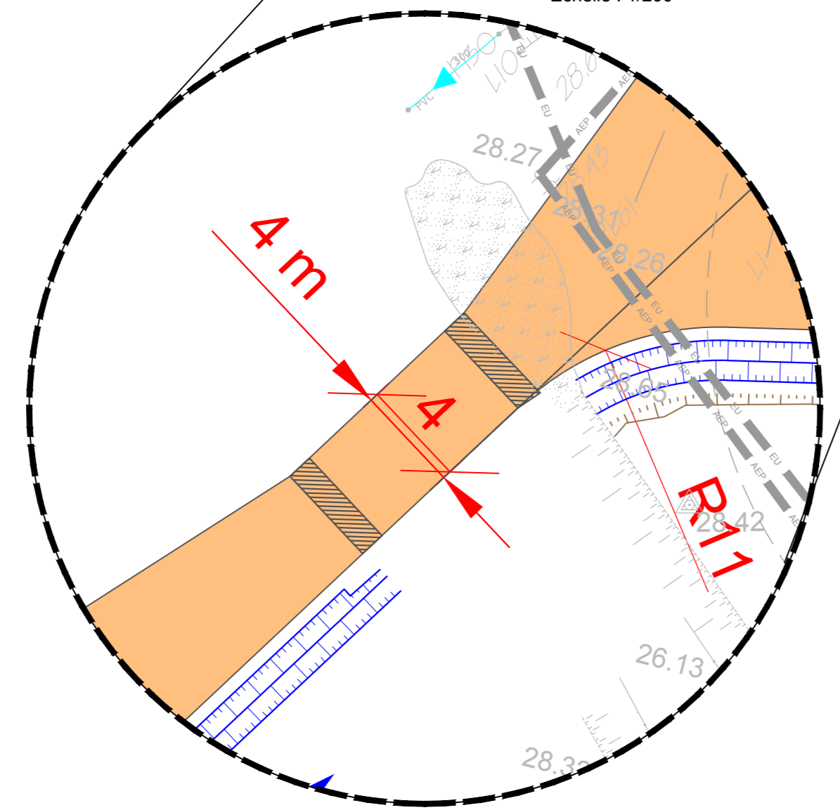
PONT PROJETE - largeur 4 m Echelle : 1/200
