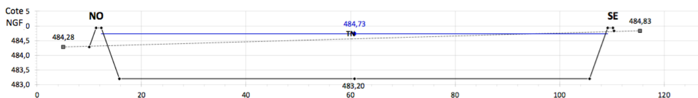
Coupe longitudinale du bassin de la serre
