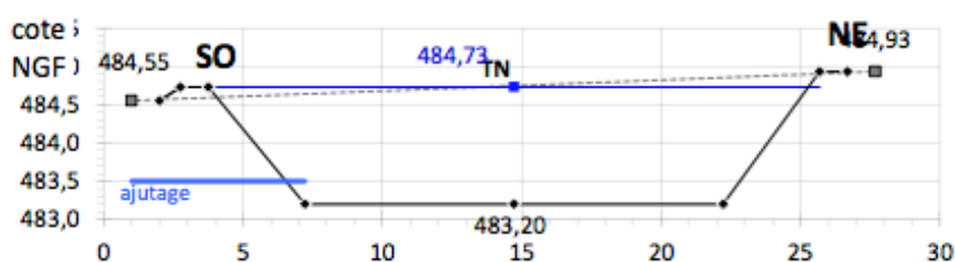
Coupe transversale du bassin de la serre
