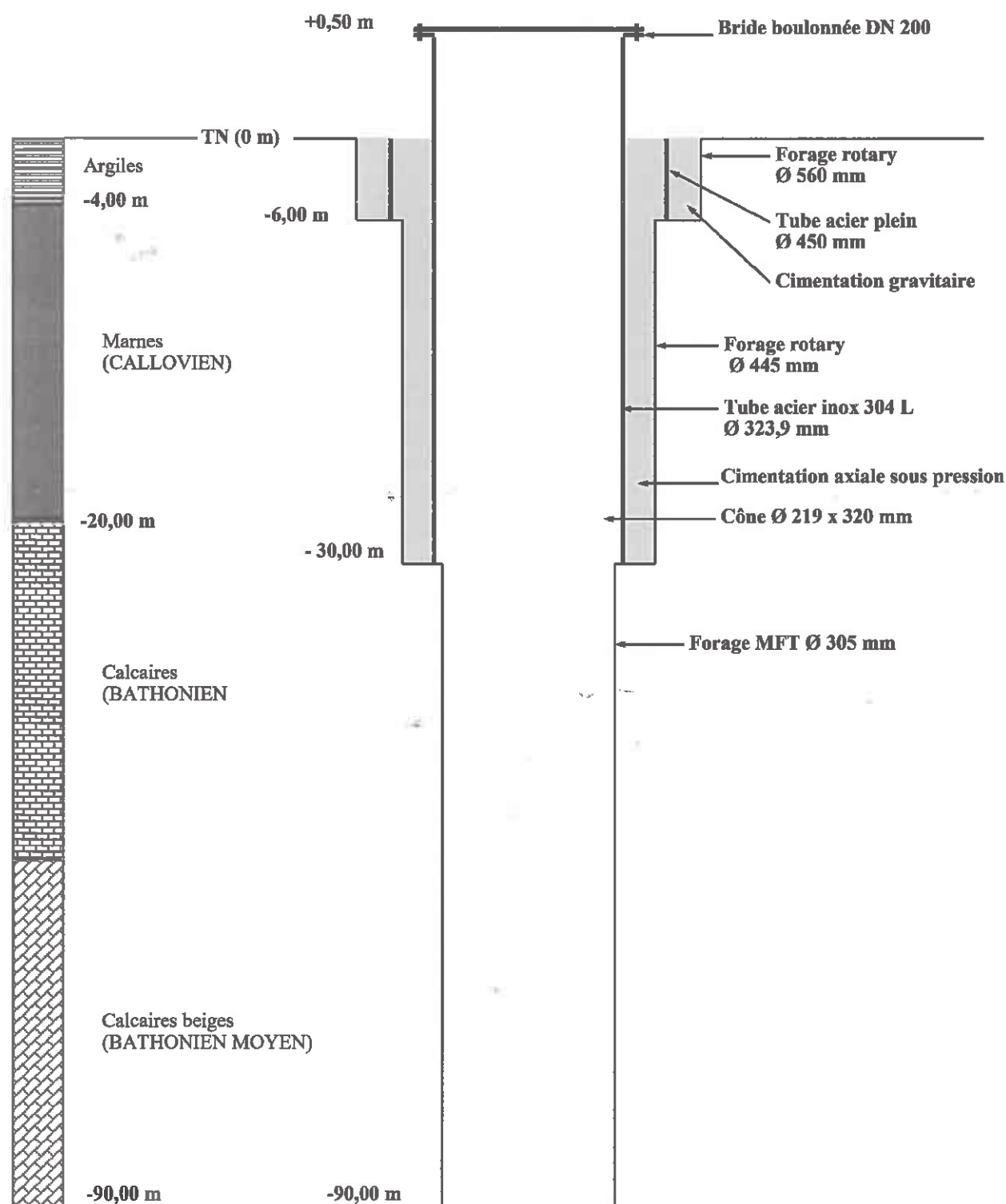
Annexe 4 : Coupe technique et géologique du forage de reconnaissance
