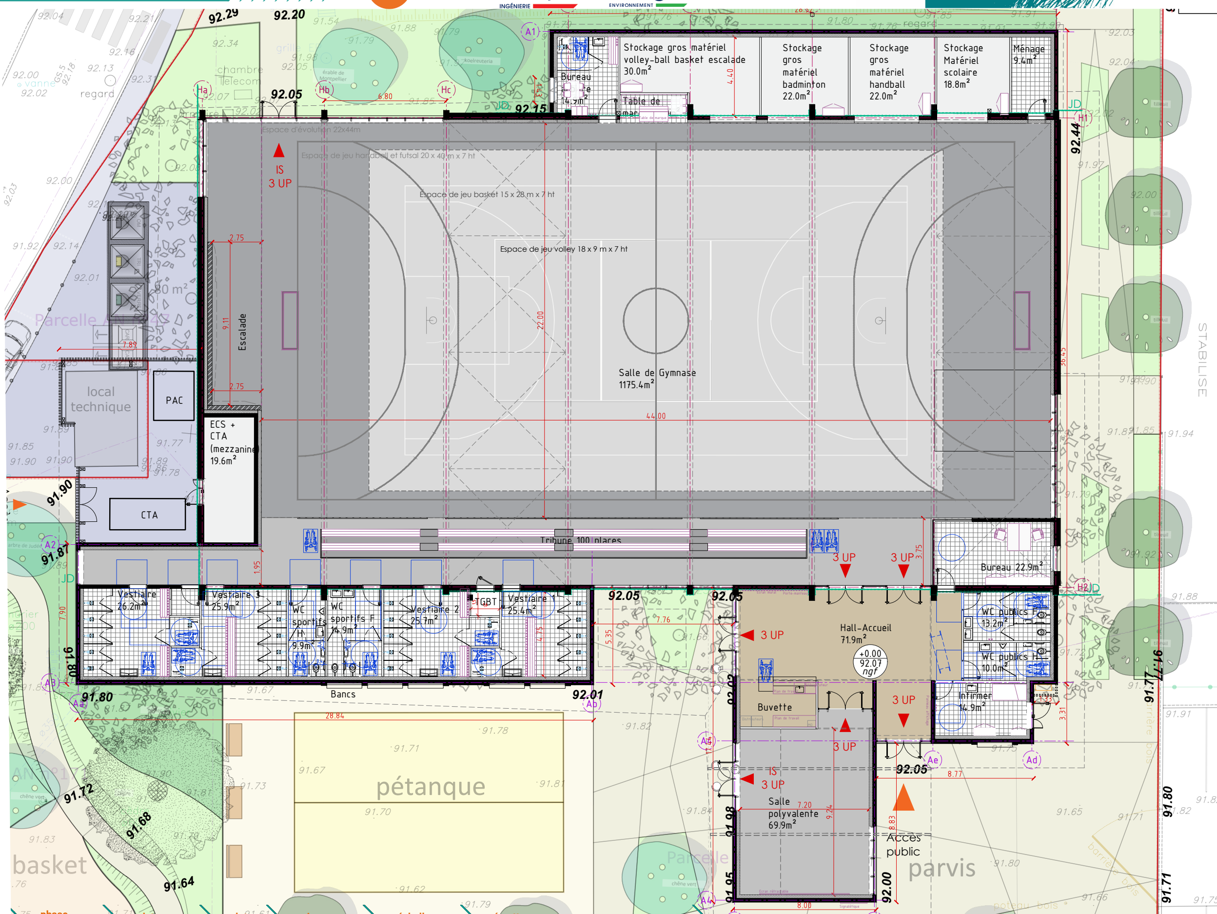
4.2 PLAN RDC 1-200
