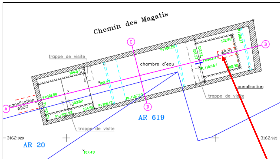
Plan topographique chambre de répartition existante
