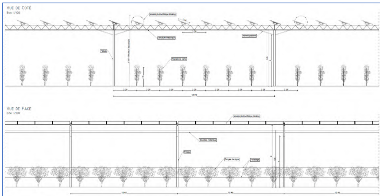
Figure 4 : Coupe longitudinale d'un rang de l'installation photovoltaïque (en m)
