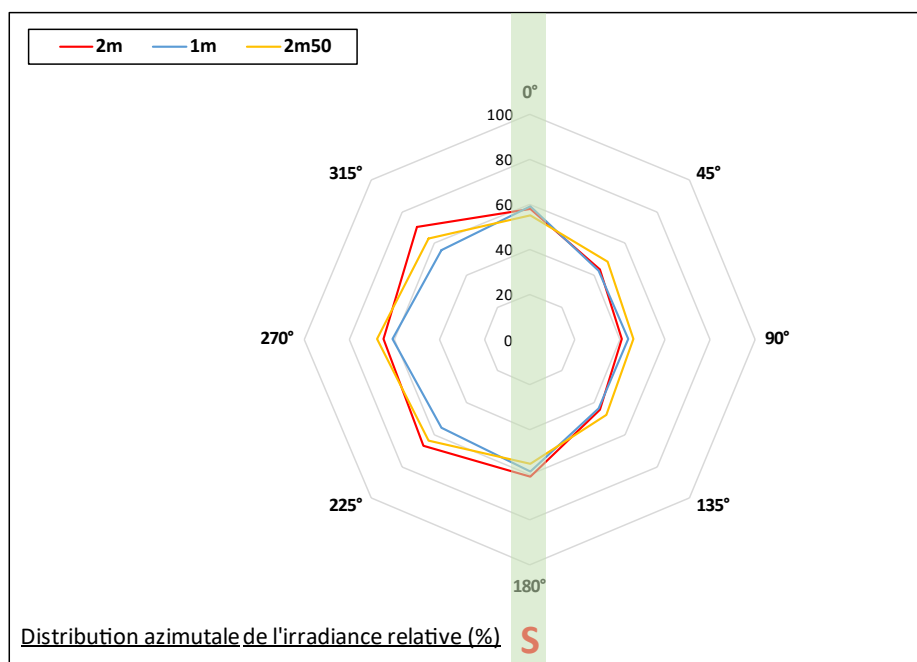
Figure 12 : Irradiance relative sous panneaux solaires simulée à 1, 2 et 2,5 m, selon l'orientation.
