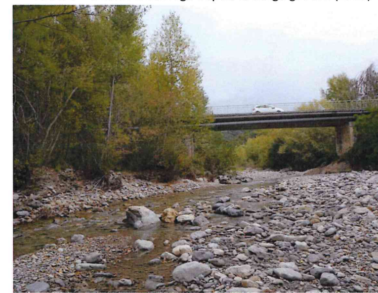
Photo 6 – Vue aval de l'ouvrage – Travée gauche (2023)
