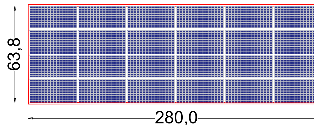
Vue Projetée - Toiture
