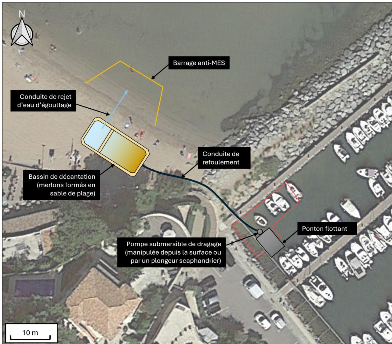
Schéma de principe des opérations de dragage d'urgence du port de Saint-Aygulf
