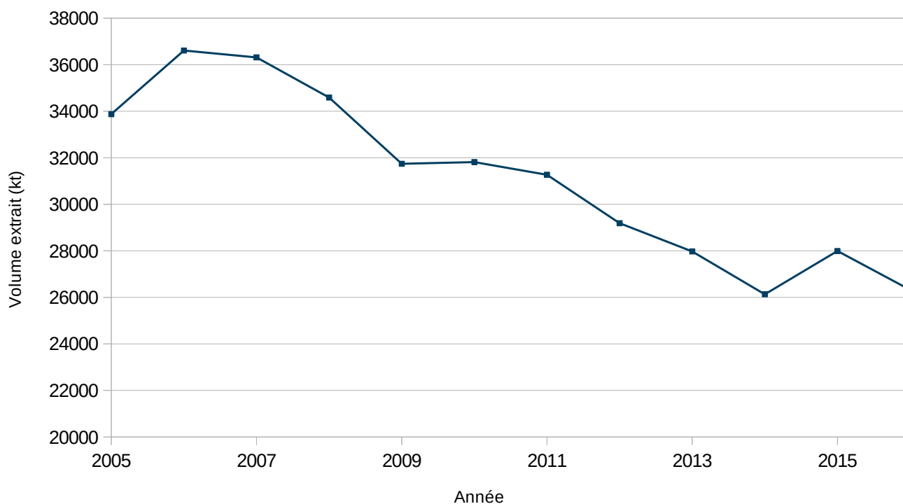
Illustration 10: Evolution des volumes extraits (toutes ressources) des carrières entre 2005 et 2015 (données issues des enquêtes annuelles « carrières » de 2005 à 2014 et de l'application GEREPA en 2015)
